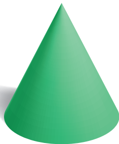
Cone
